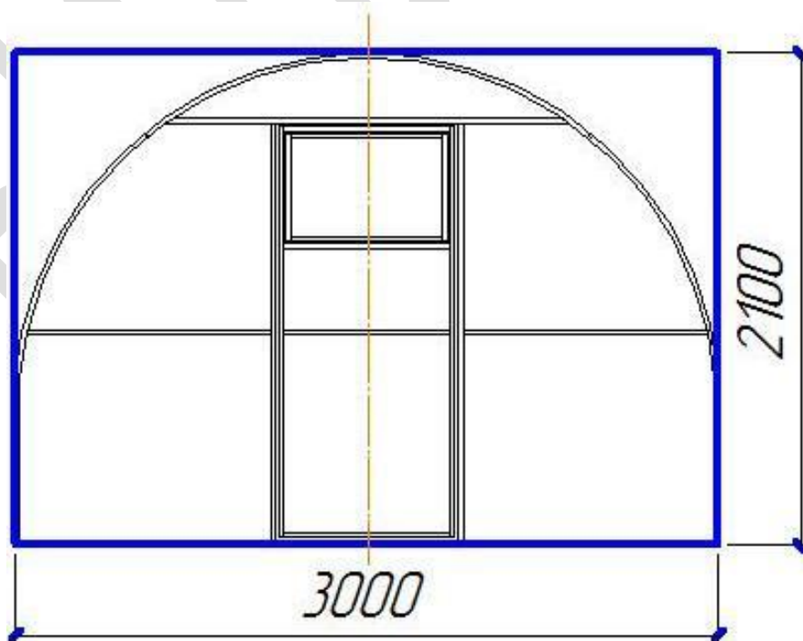
Рис. 5. Схема раскроя поликарбоната на торцы теплицы.
