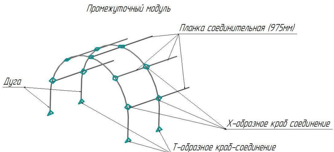
Рис.3 Схема сборки модулей каркаса теплицы «Апрель»
