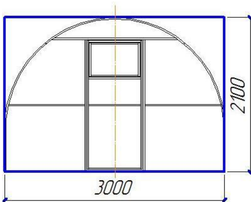
Рис. 5. Схема раскроя поликарбоната на торцы теплицы.
