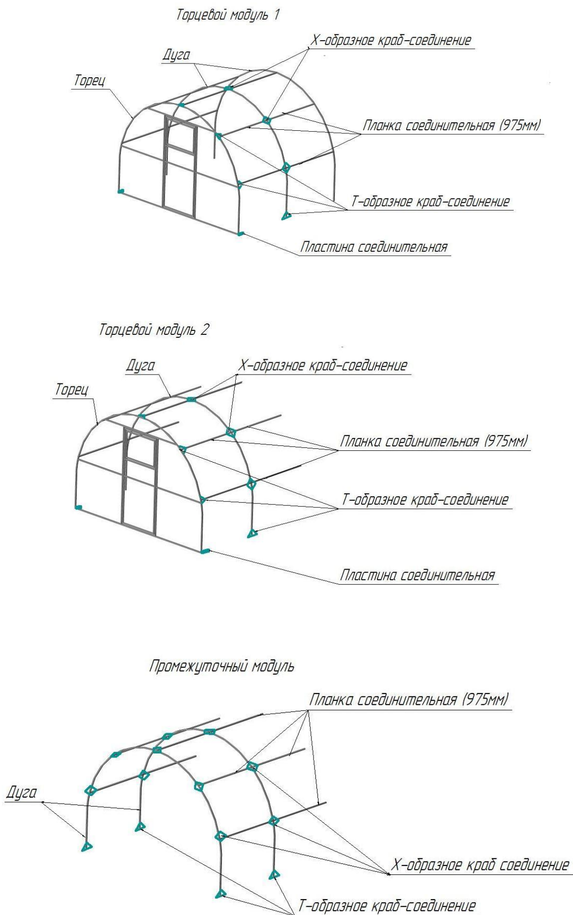
Рис.3 Схема сборки модулей каркаса теплицы «Апрель»
